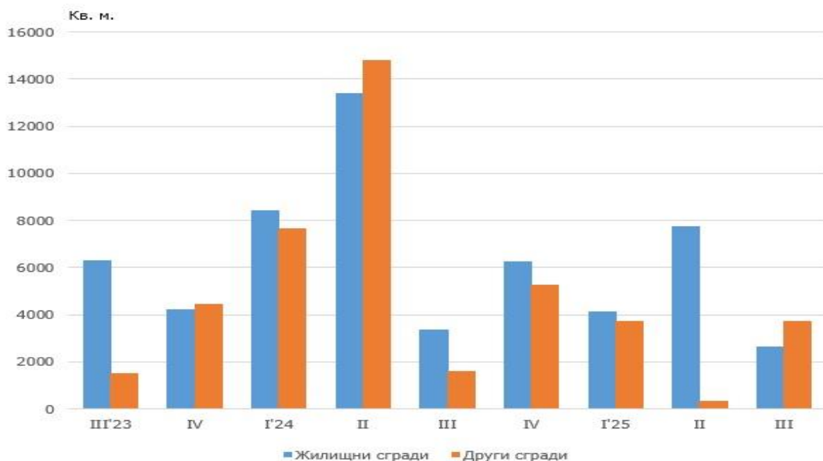
Фиг.2. Издадени разрешителни за строеж - разгъната застроена площ в област Търговище по видове сгради и по тримесечия
