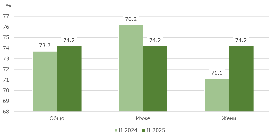
Фиг.1. Коефициенти на заетост за възрастовата група 15 - 64 навършени години в област Благоевград по пол през второто тримесечие на 2024 и 2025 година
