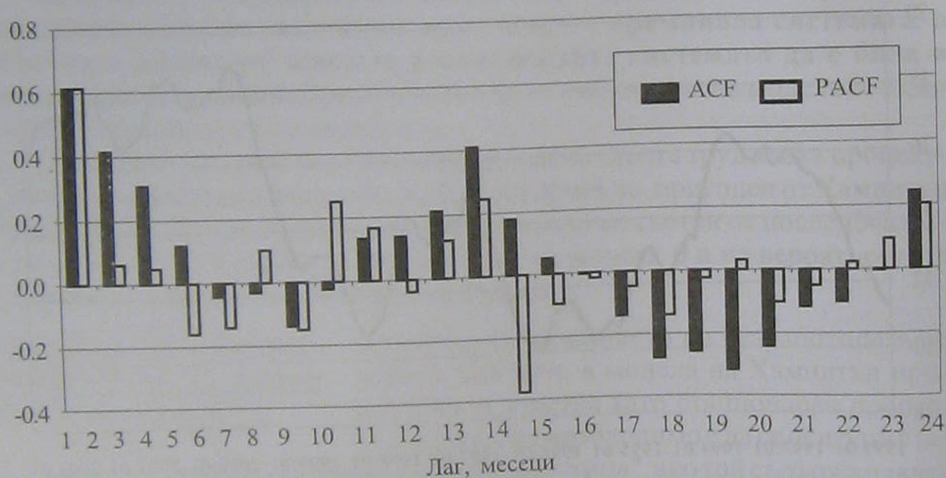
Фиг. 3. Автокорелационни (ACF) и частни автокорелационни (PACF) коефициенти за първите разлики на динамичния ред на равнището на безработицата
