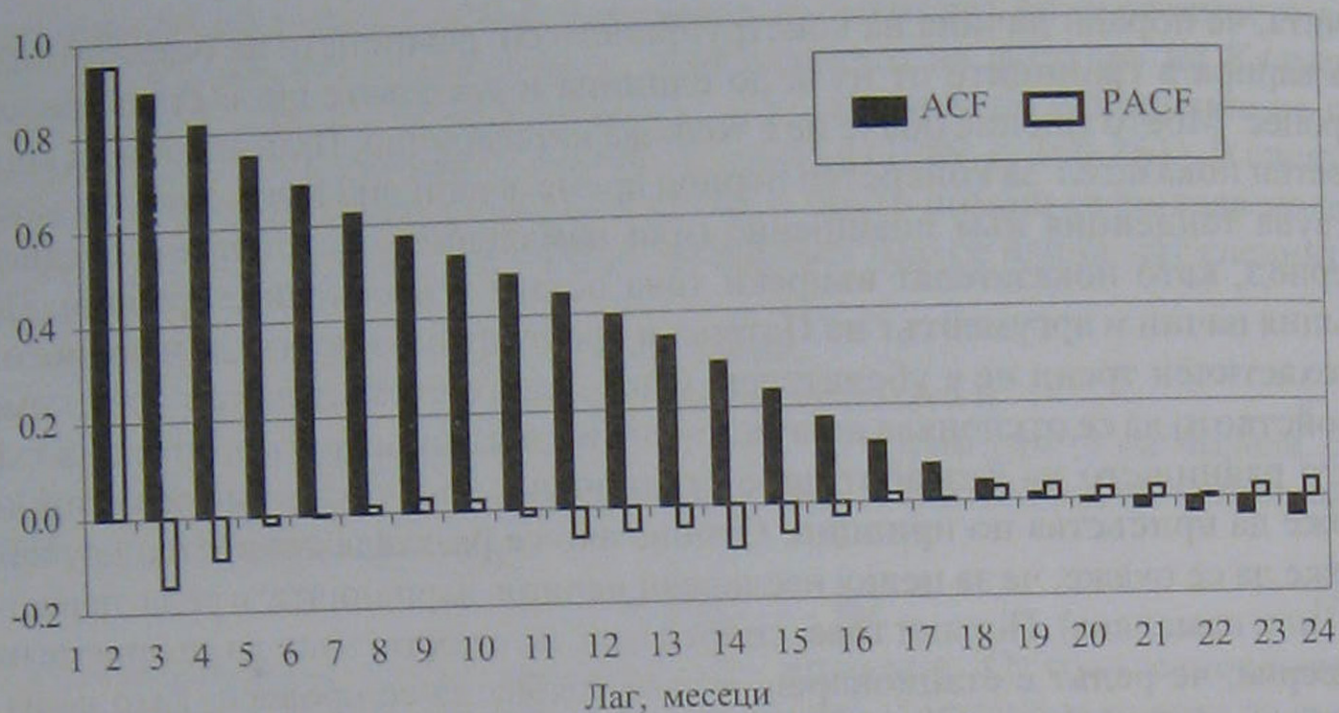
Фиг. 2. Автокорелационни (ACF) и частни автокорелационни (PACF) коефициенти за динамичния ред на равнището на безработицата
