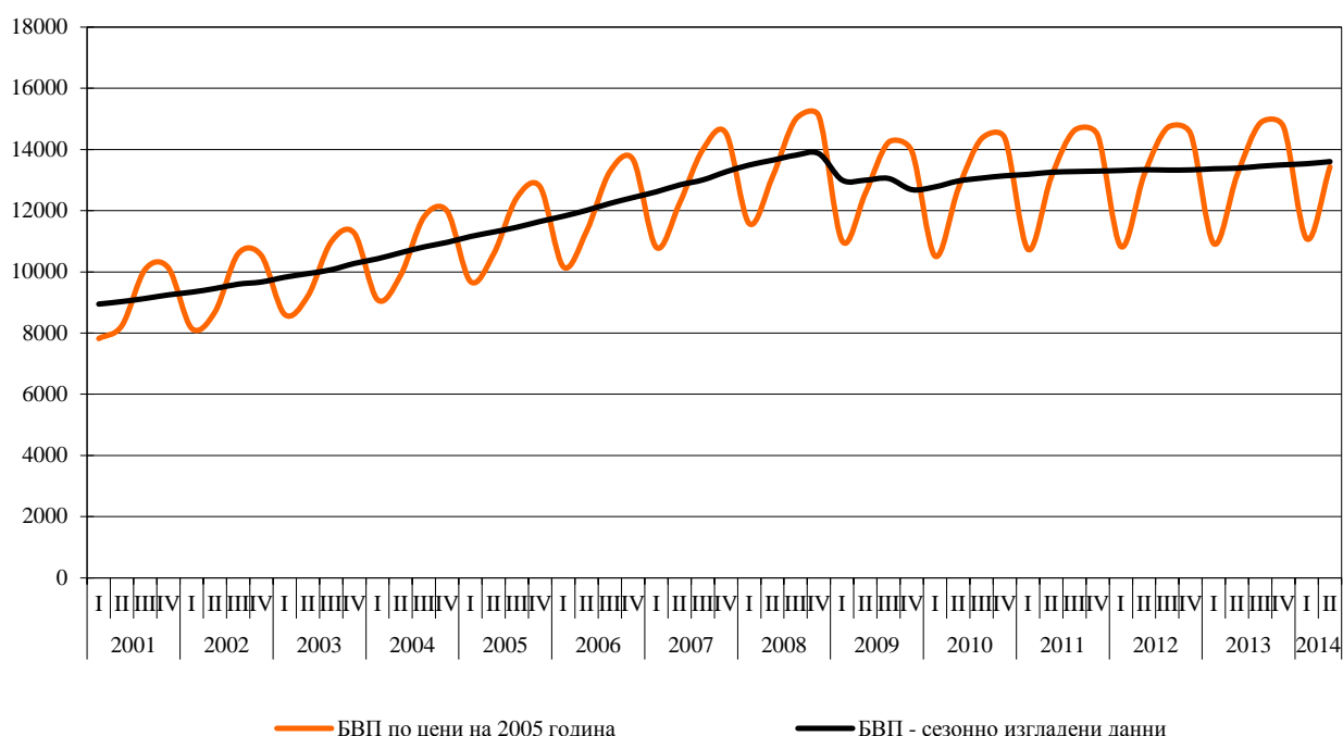
Фиг. 1. БВП по тримесечия за периода 2001 - 2014 г. по средногодишни цени на 2005 година
