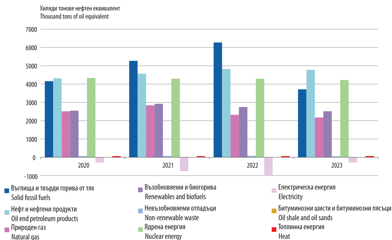
Фиг. 25. Брутно вътрешно потребление Figure 25. Gross inland consumption
