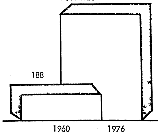
ЖЕЛЕЗНИ РУДИ /съдържание на желязо/ хил.тонове
