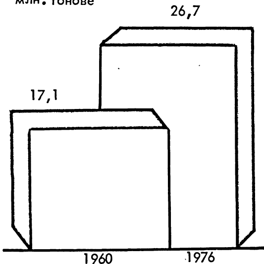
ДОБИВ НА КАМЕННИ ВЪГЛИЩА млн. тонове
